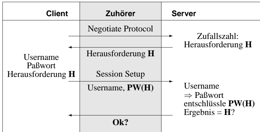
Abbildung 8: Challenge-Response Verfahren
