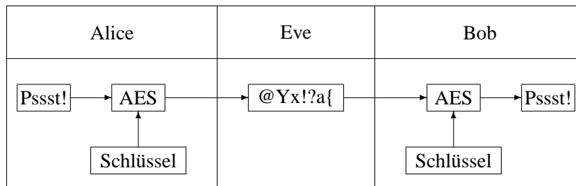
Abbildung 6: Symmetrische Verschlüsselung
